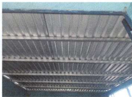
Foto 1: Sustitución de lámina por lámina troquelada aluzinc calibre 26, susustitución de soporte de madera por soporte de metal y sustitución de elementos de fijación en la cocina.
